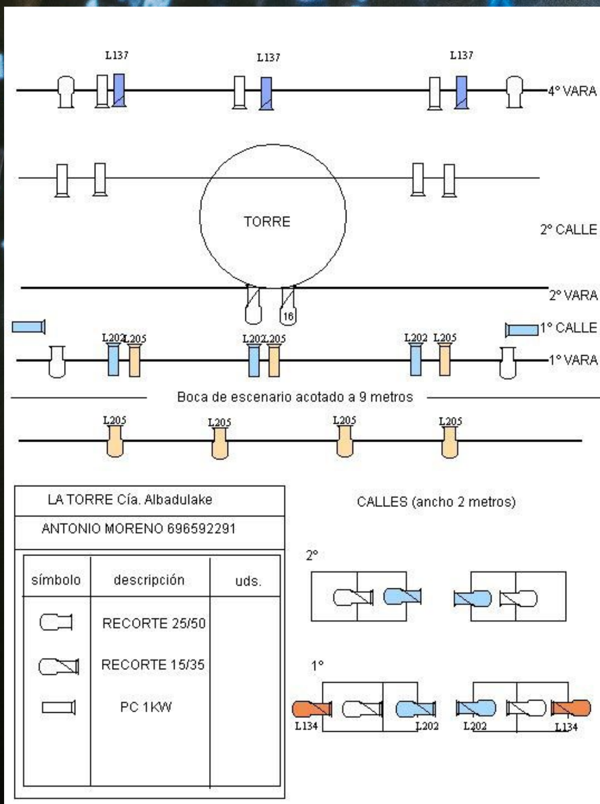
[PLANO DE LUCES]
